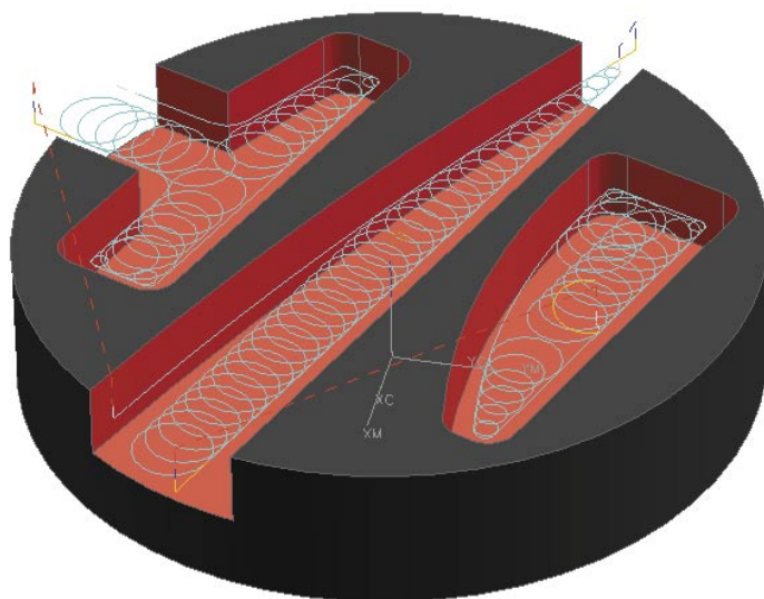
Rys. 4. Prowadzenie wydajnej obróbki HSM jest umożliwiające m.in. dzięki optymalizowaniu ścieżek narzędzi obróbczych
