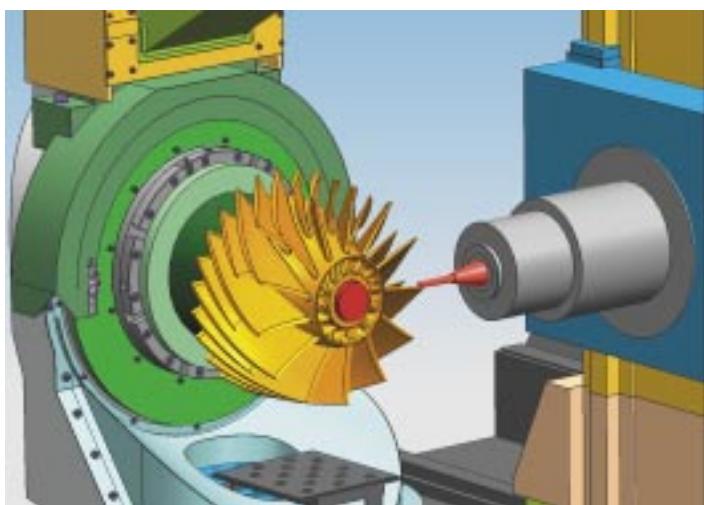
Rys. 3. Przykład symulacja obróbki 5-osiowej, generowanej w NX CAM Express
