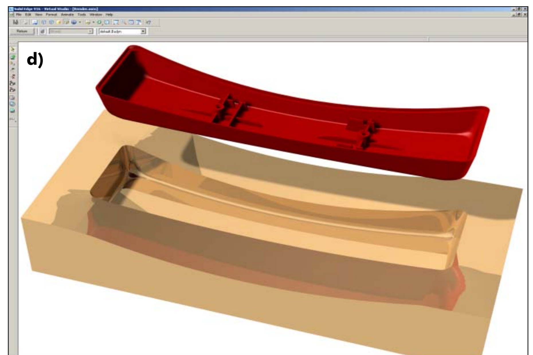
Rys. 1. Symulacja CAM frezowania matrycy: a) obróbka zgrubna, b) półwykańczająca, c) wykańczająca, d) gotowa matryca
