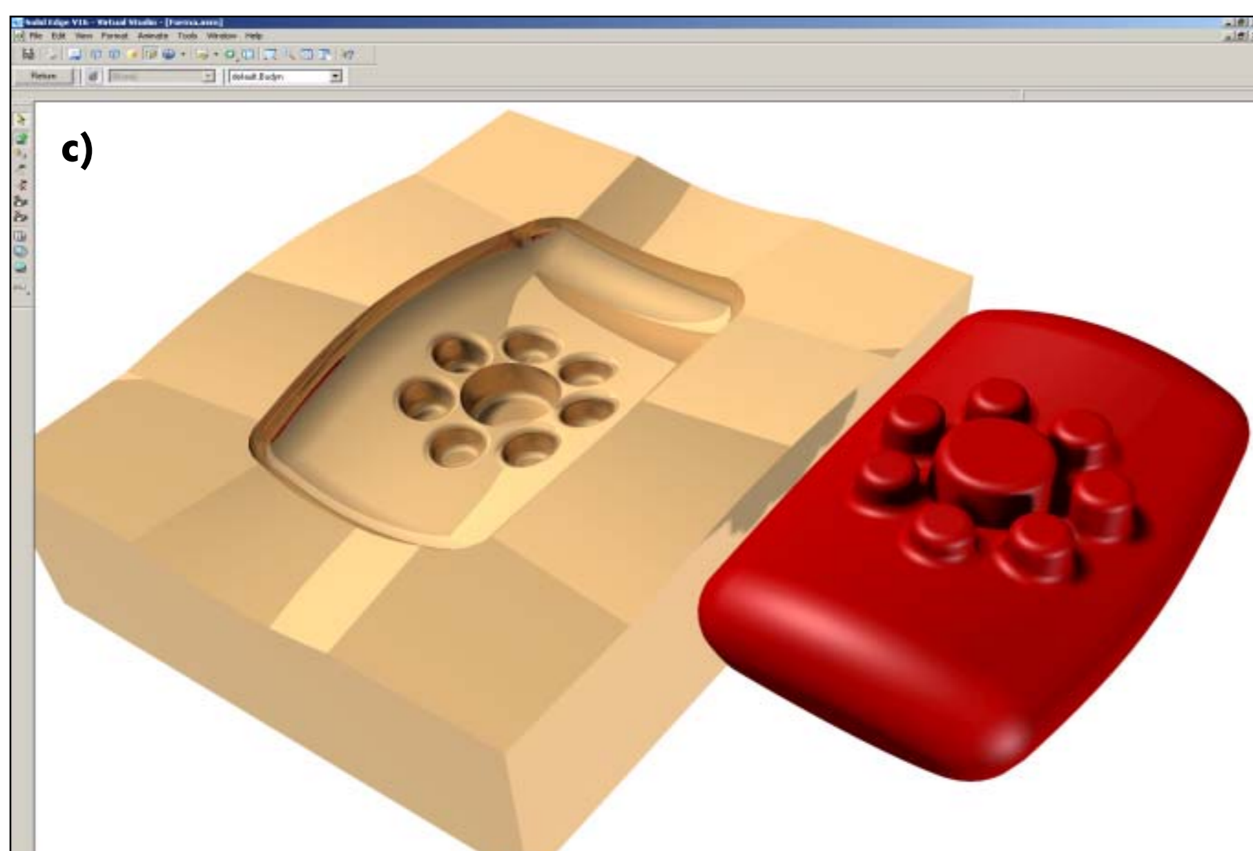
Rys. 2. Automatyczna aktualizacja ścieżki narzędzia CAM (NX2) w wyniku zmiany wejściowej geometrii CAD (SEV16): a) geometria początkowa, b) zdefiniowana obróbka – frezowanie półwykańczające, c) zmieniona geometria, d) obróbka zaktualizowana
